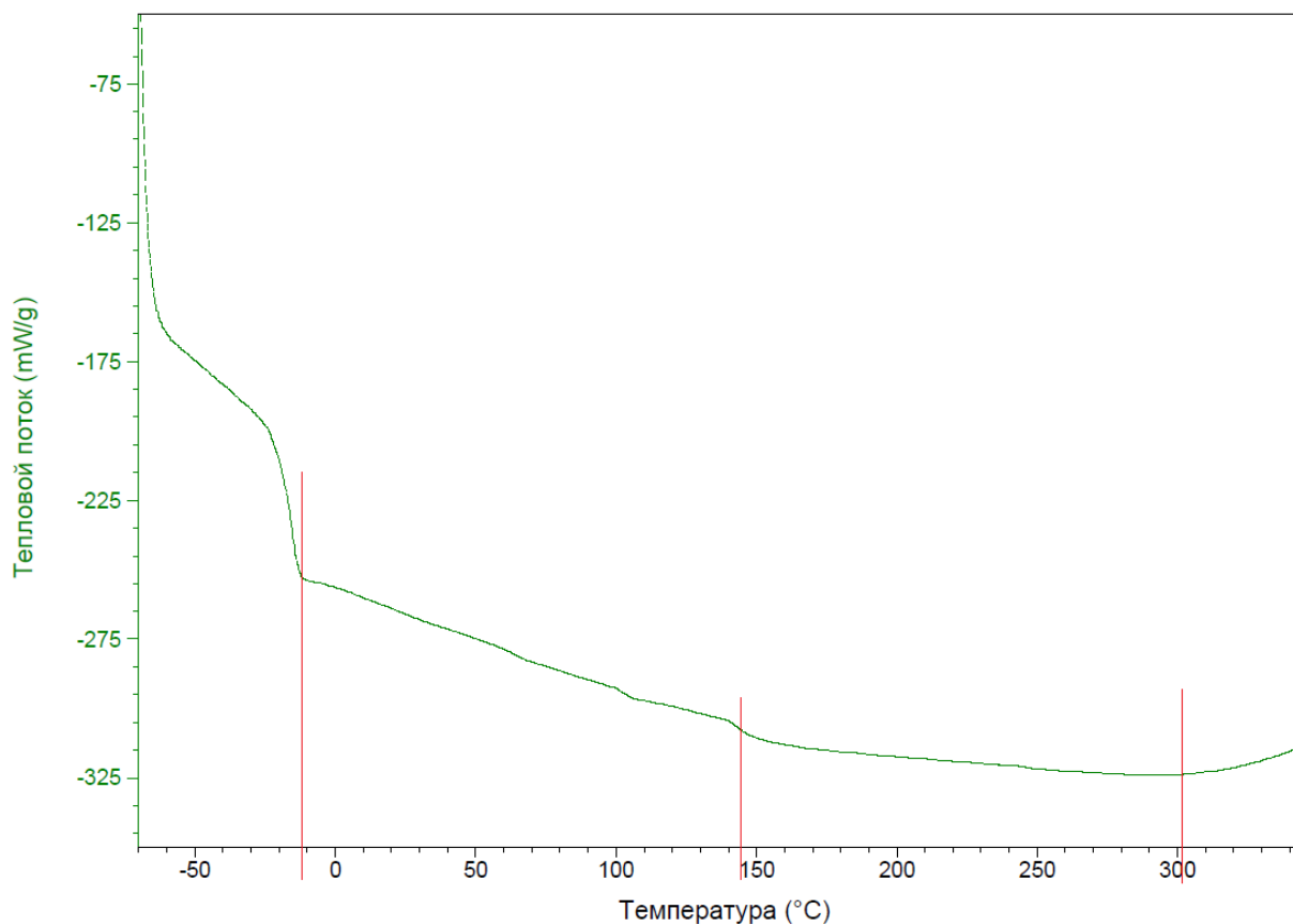
Рисунок 1 – Графік ДСК зразка 00-00-00-0
