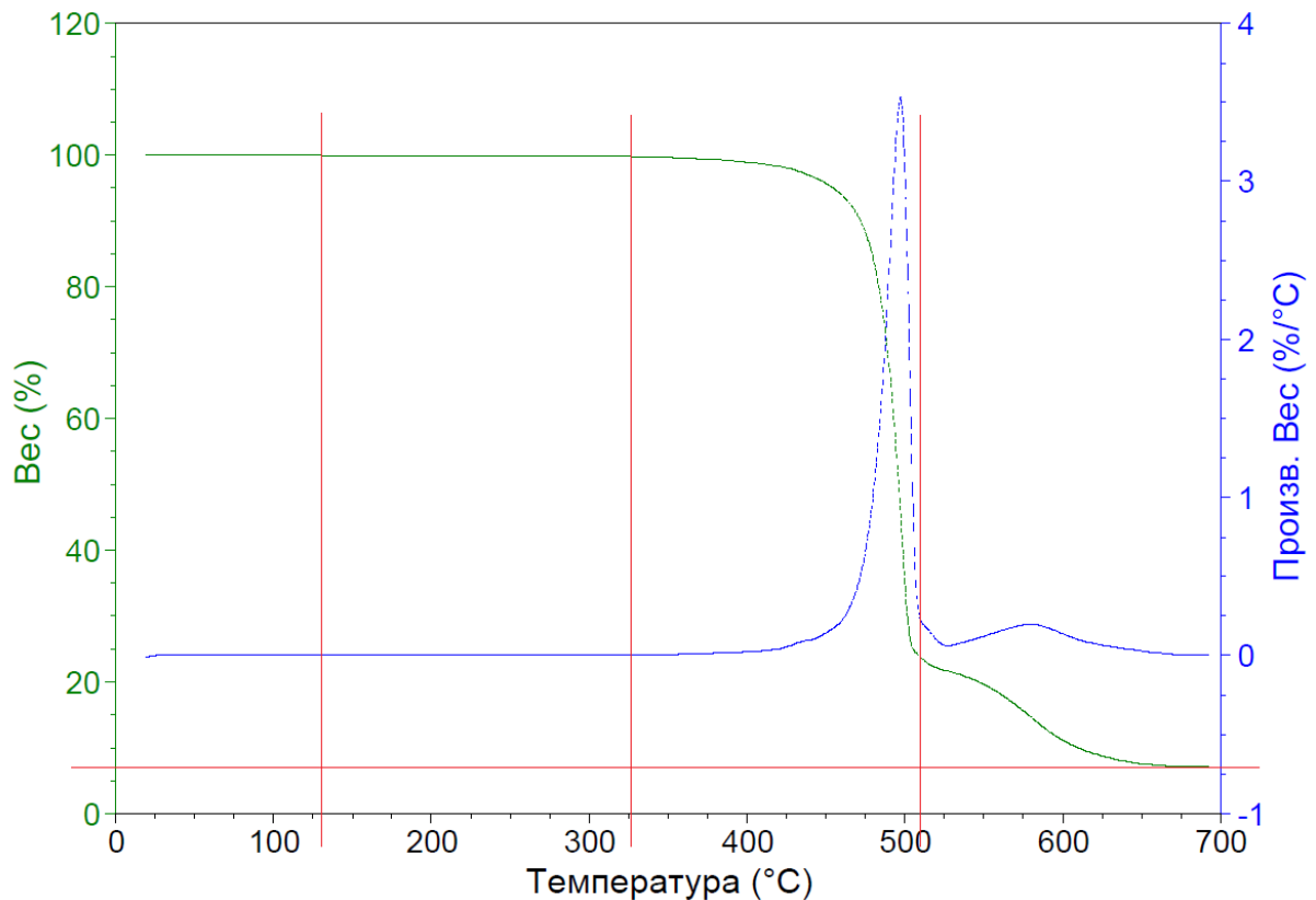
Рисунок 2 – Графік ТГА зразка 00-00-00-0
