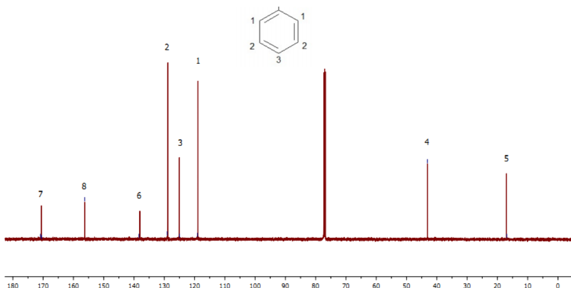
Рисунок 6 – Аналіз отриманого спектру NMR-13C зразка 1
