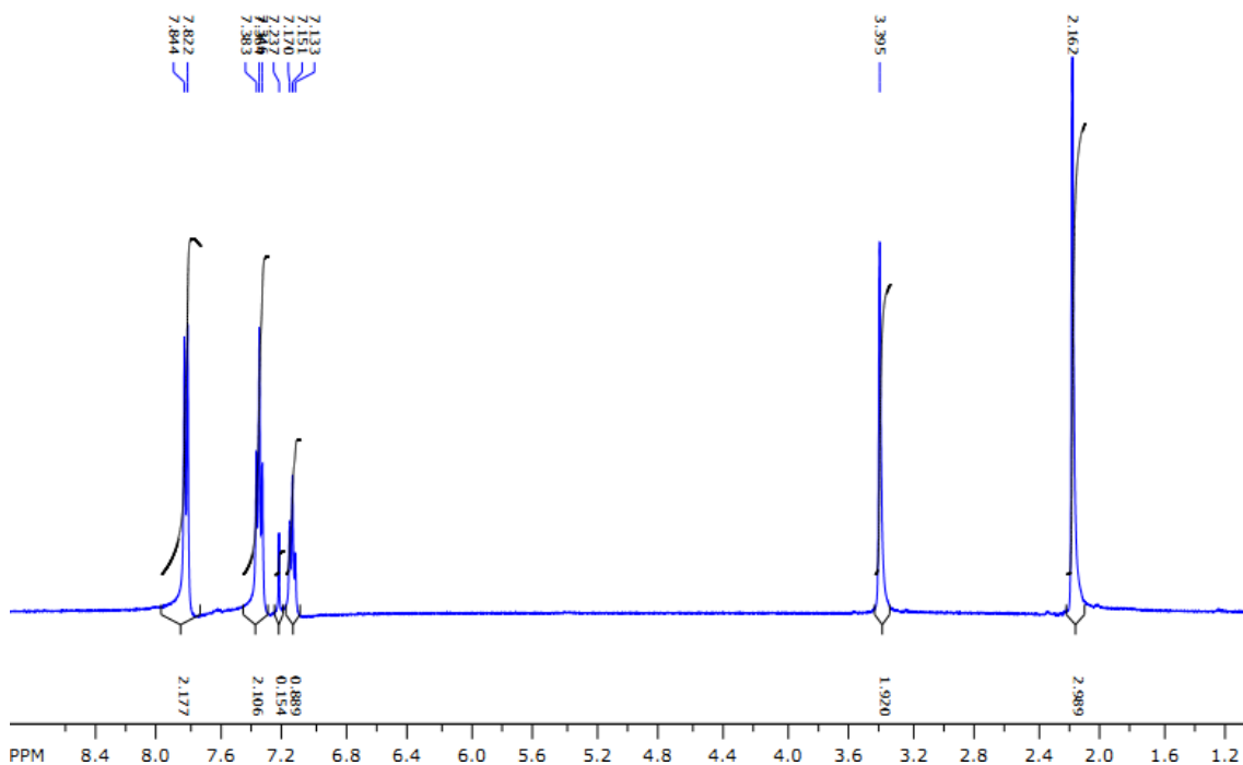
Рисунок 1 – Спектрограма PMR зразка 1
