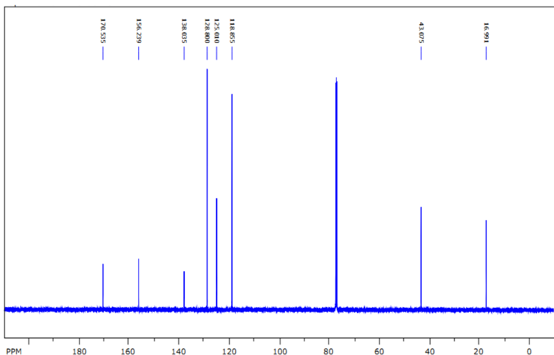
Рисунок 5 – Спектрограма NMR-13C зразка 1
