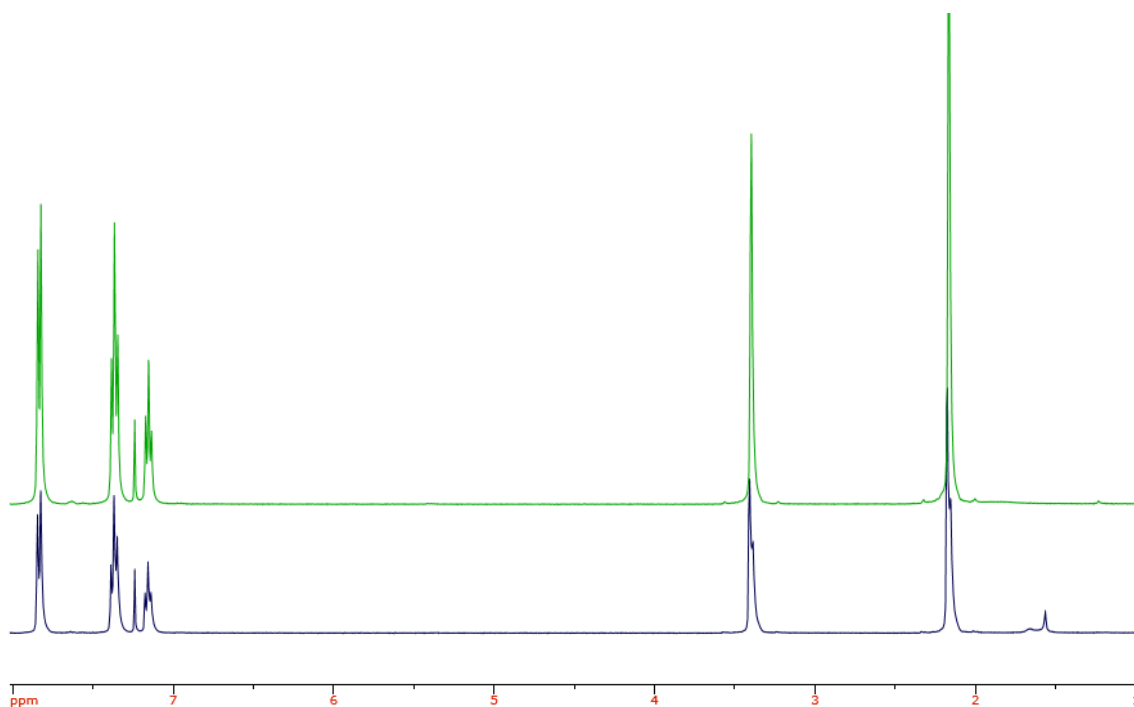
Рисунок 4 – Накладання спектрів зразків 1 (зелений) та 2 (синій)
