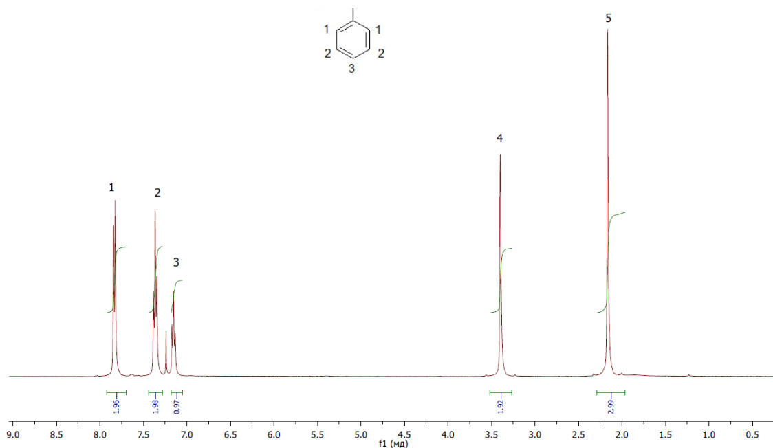
Рисунок 2 – Аналіз отриманого спектру PMR зразка 1
