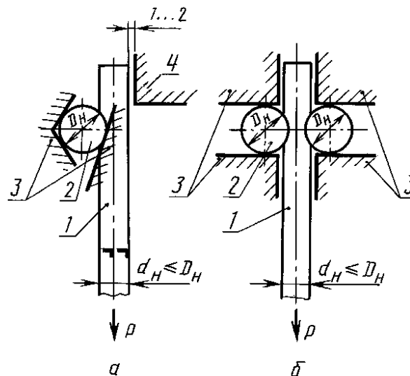
Схемы испытаний крестообразных соединений на срез
