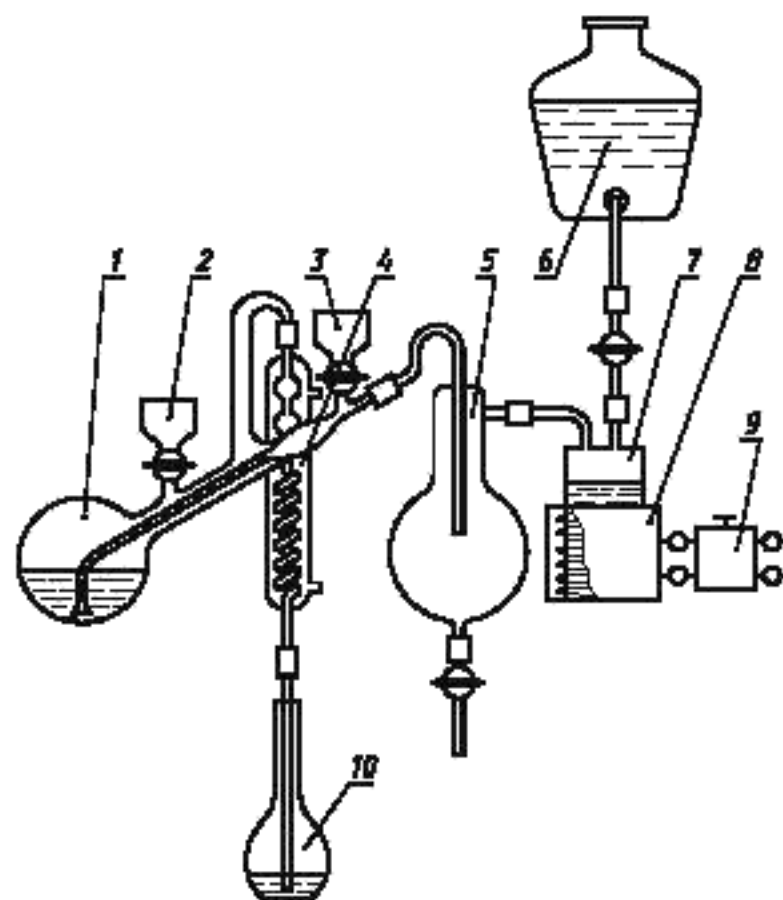
Рисунок 1 — Схема установки для дистилляции аммиака с паром
