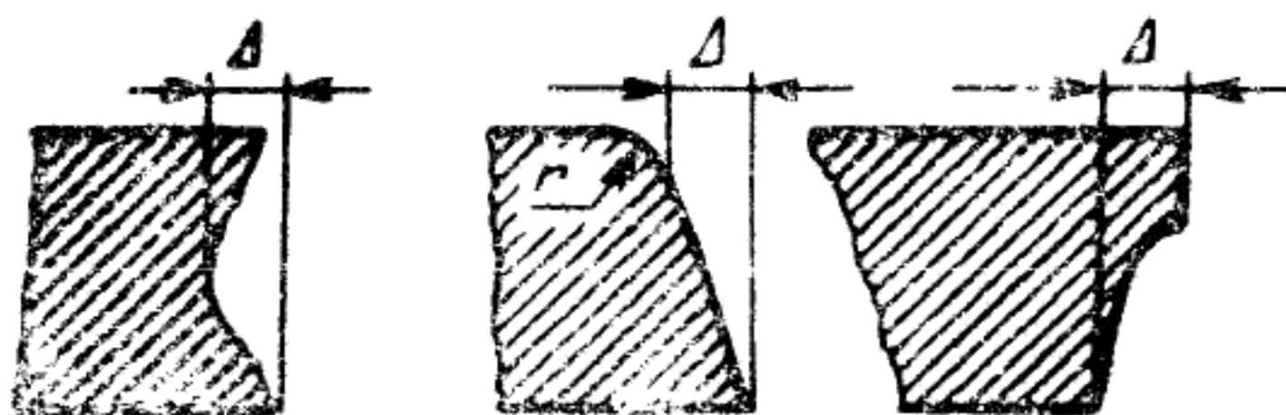
Δ — отклонение поверхности реза от перпендикулярности
