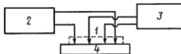
Блок-схема установки для измерения удельного электрического сопротивления
