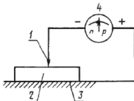
1 - зонд; 2 - образец; 3 - металлическая пластина; 4 - нуль-индикатор
