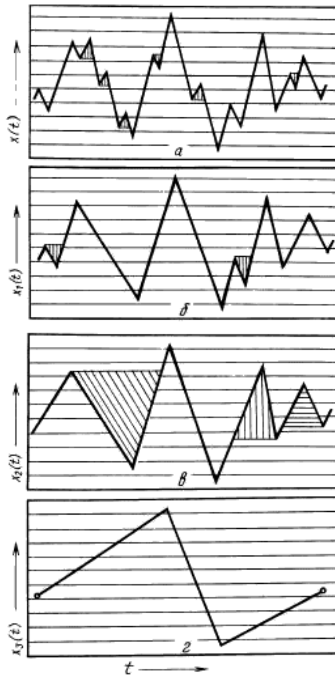
Схематизация по методу полных циклов
