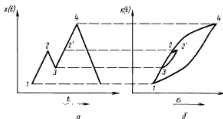
а — фрагмент процесса нагружения; б — диаграмма «напряжение—деформация»
