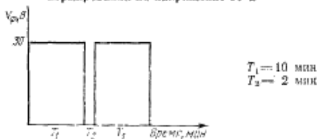
Схема формовки образцов при нормировании на напряжение 30 В
