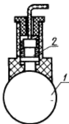
1 — объект контроля; 2 — преобразователь вихретокового измерителя
