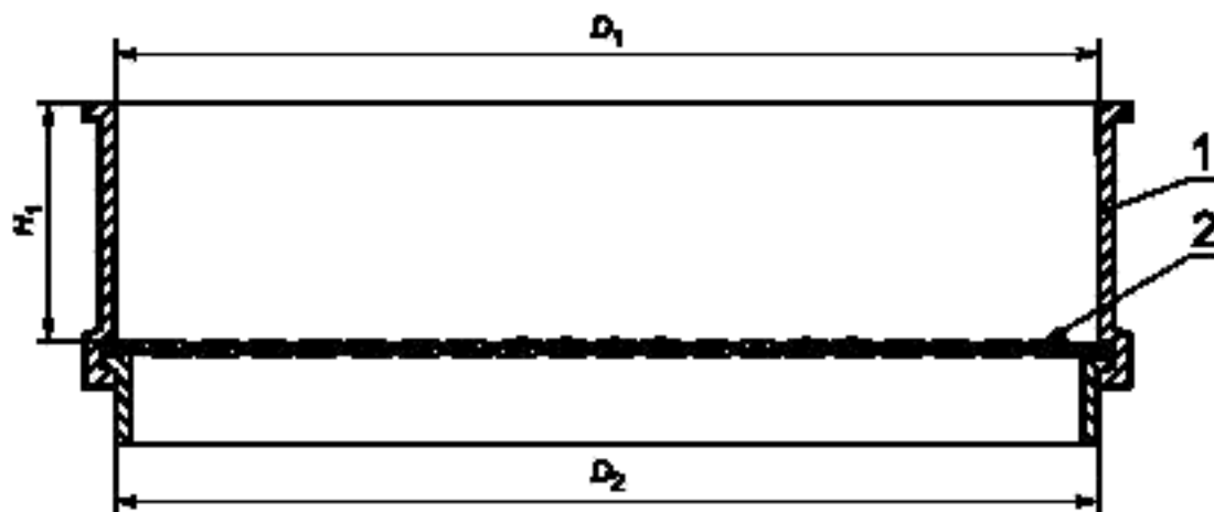
1 — обечайка (рамка); 2 — сетка из металлической проволоки
